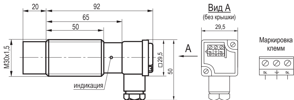
Габаритный чертеж
