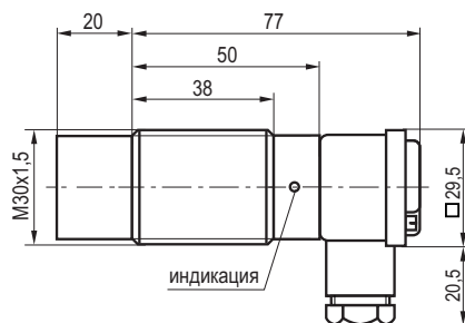
Габаритный чертеж
