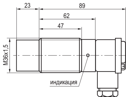
Габаритный чертеж
