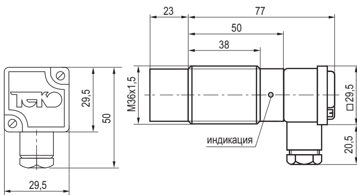
Габаритный чертеж
