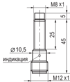
Габаритный чертеж
