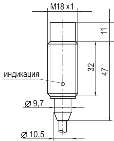
Габаритный чертеж
