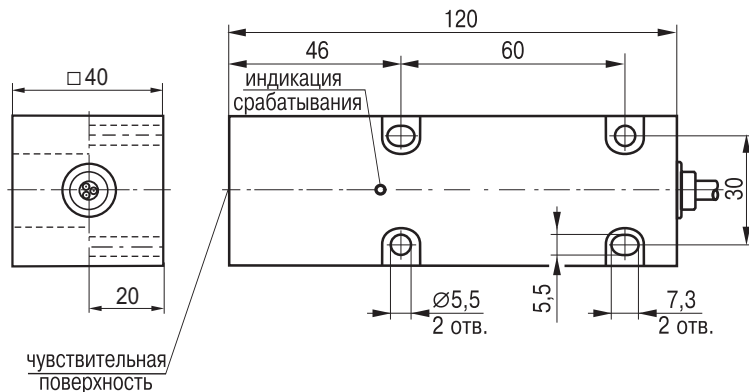
Габаритный чертеж
