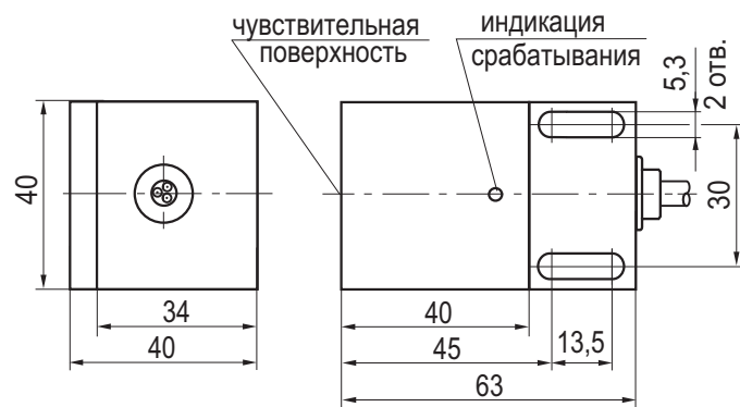
Габаритный чертеж
