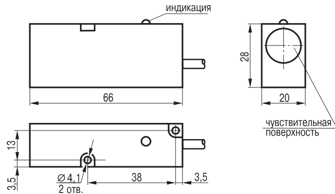
Габаритный чертеж
