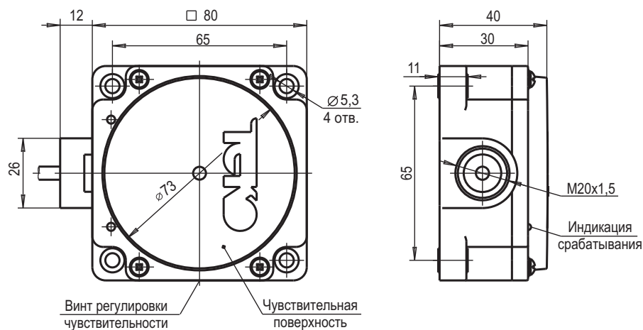
Габаритный чертеж
