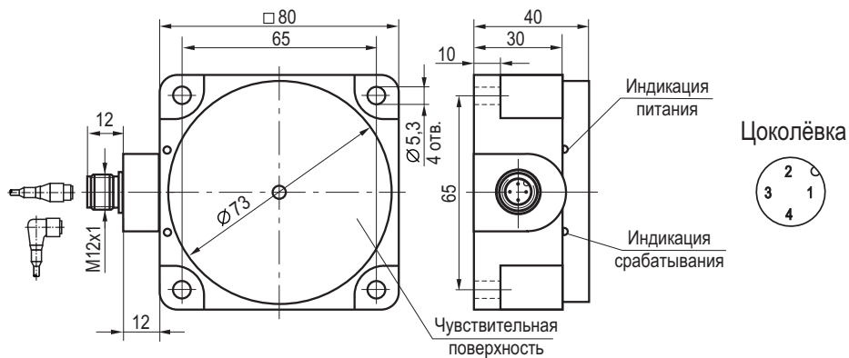
Габаритный чертеж
