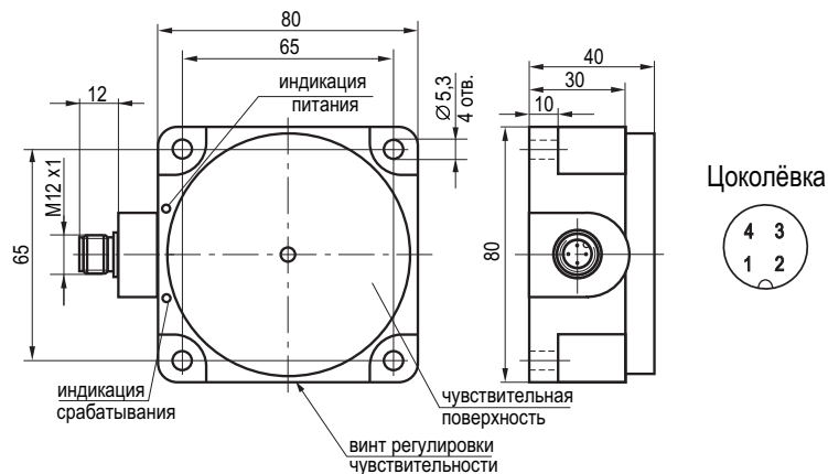
Габаритный чертеж
