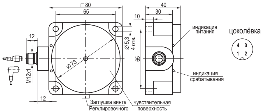
Габаритный чертеж
