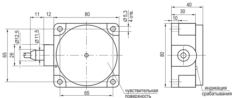
Габаритный чертеж
