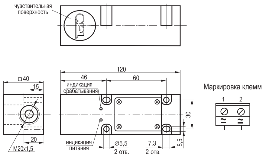
Габаритный чертеж
