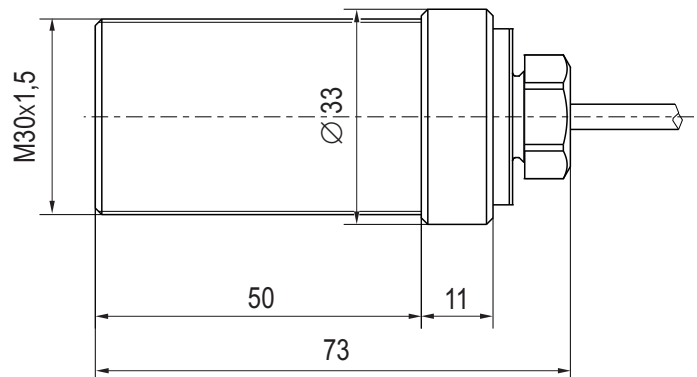
Габаритный чертеж
