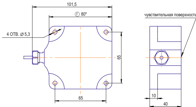
Габаритный чертеж
