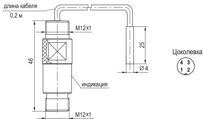
Габаритный чертеж
