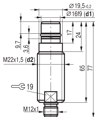
Габаритный чертеж
