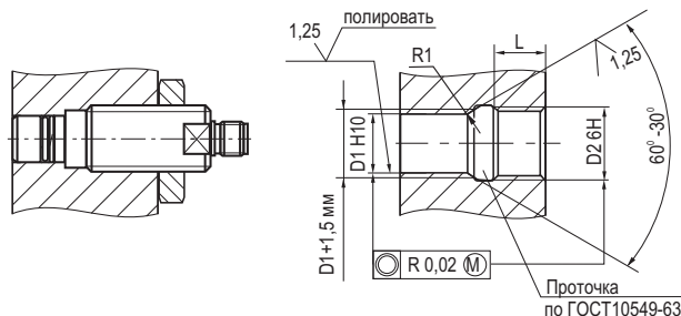
Схема монтажа
