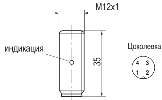
Габаритный чертеж
