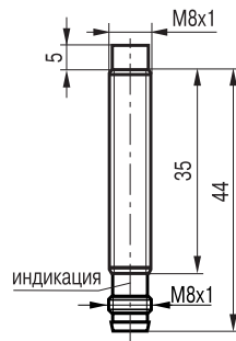
Габаритный чертеж
