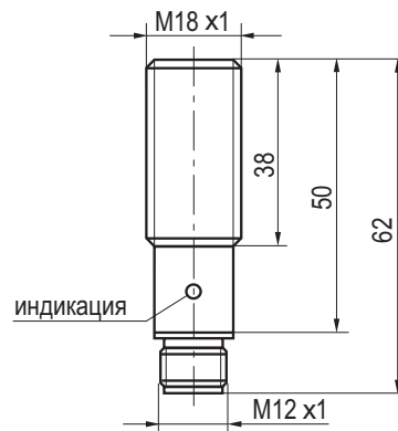
Габаритный чертеж
