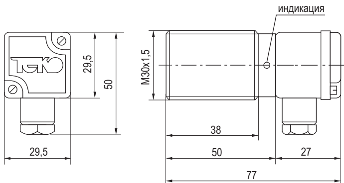
Габаритный чертеж
