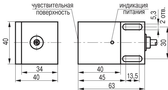
Габаритный чертёж
