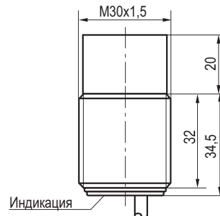
Габаритный чертеж
