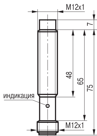
Габаритный чертеж
