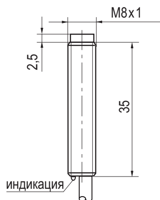
Габаритный чертеж
