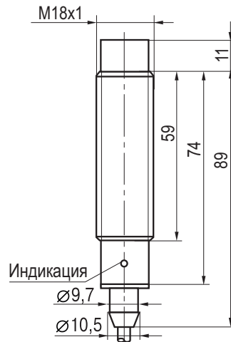
Габаритный чертеж
