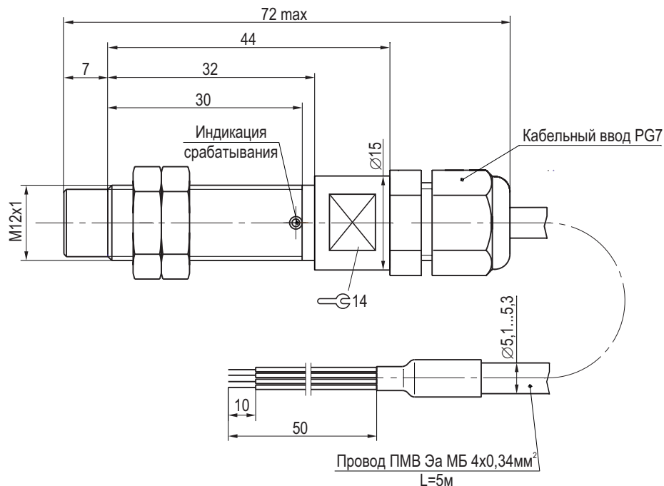
Габаритный чертеж
