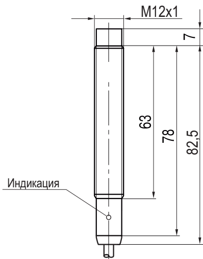
Габаритный чертеж
