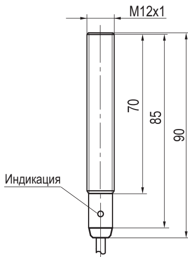
Габаритный чертеж
