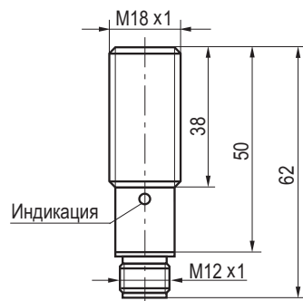
Габаритный чертеж
