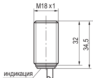
Габаритный чертеж
