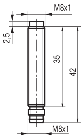
Габаритный чертеж
