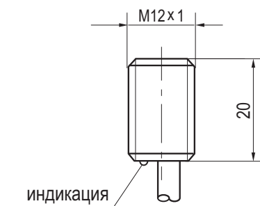
Габаритный чертеж
