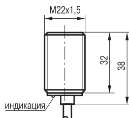
Габаритный чертеж
