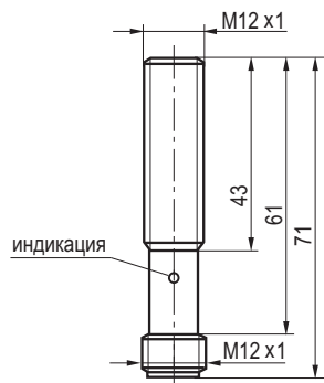
Габаритный чертеж
