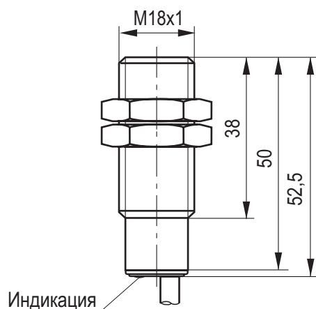
Габаритный чертёж
