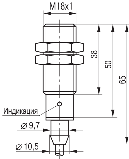
Габаритный чертеж
