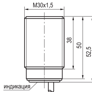
Габаритный чертеж
