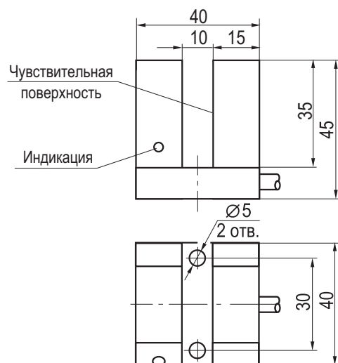
Габаритный чертеж
