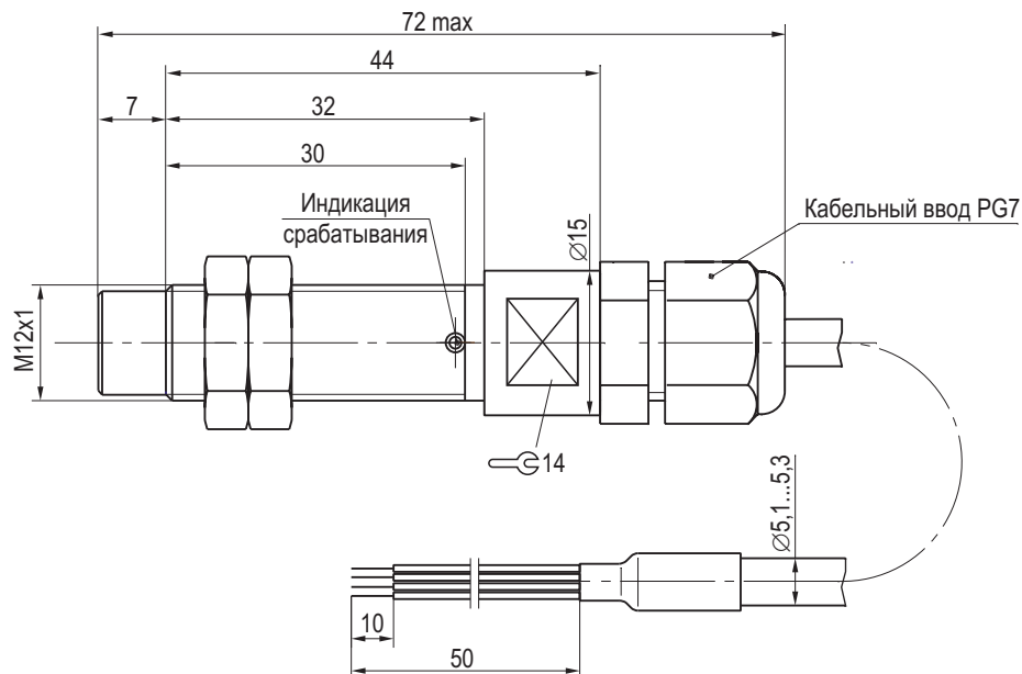
Габаритный чертёж
