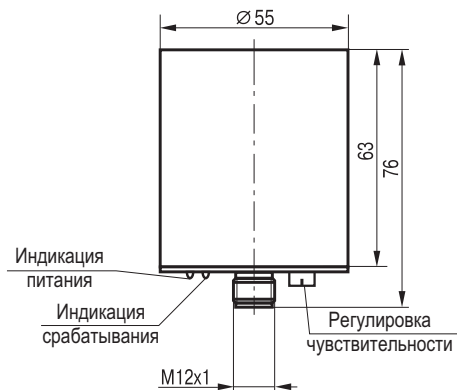
Габаритный чертеж
