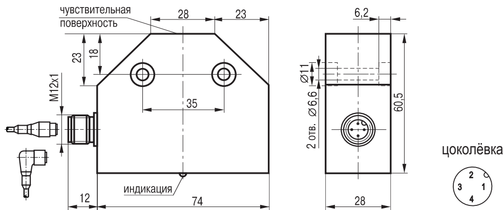
Габаритный чертеж
