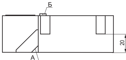
Габаритный чертеж
