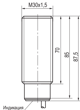
Габаритный чертеж
