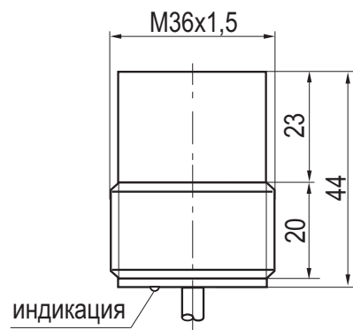
Габаритный чертеж
