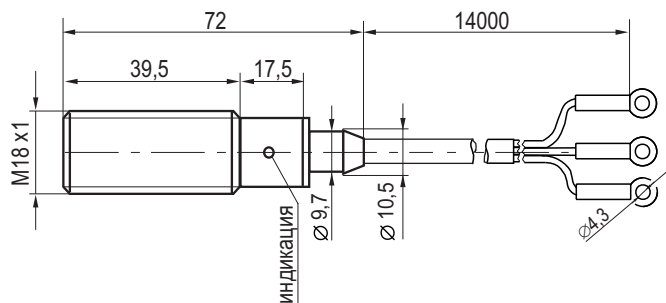
Габаритный чертеж
