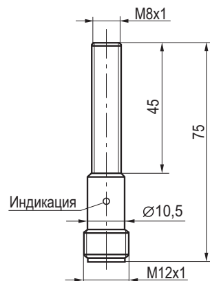
Габаритный чертеж
