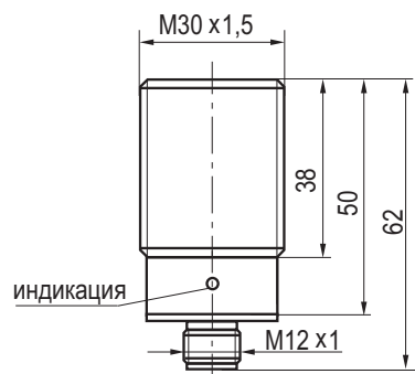
Габаритный чертеж
